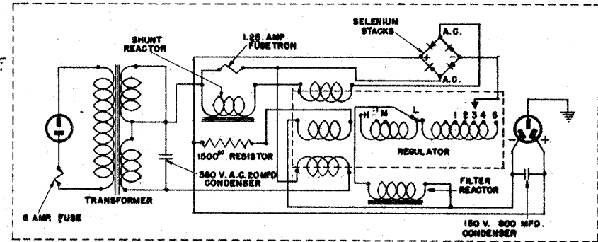
SCHEMATIC WIRING
